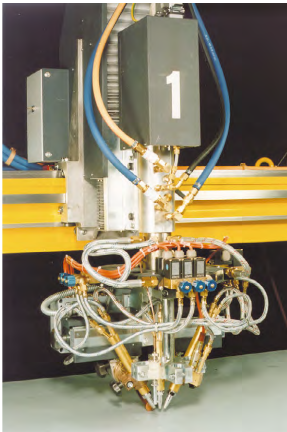
Głowica trójpalnikowa, ukosująca IR (o nieskończonej rotacji, nastawy ręczne)
