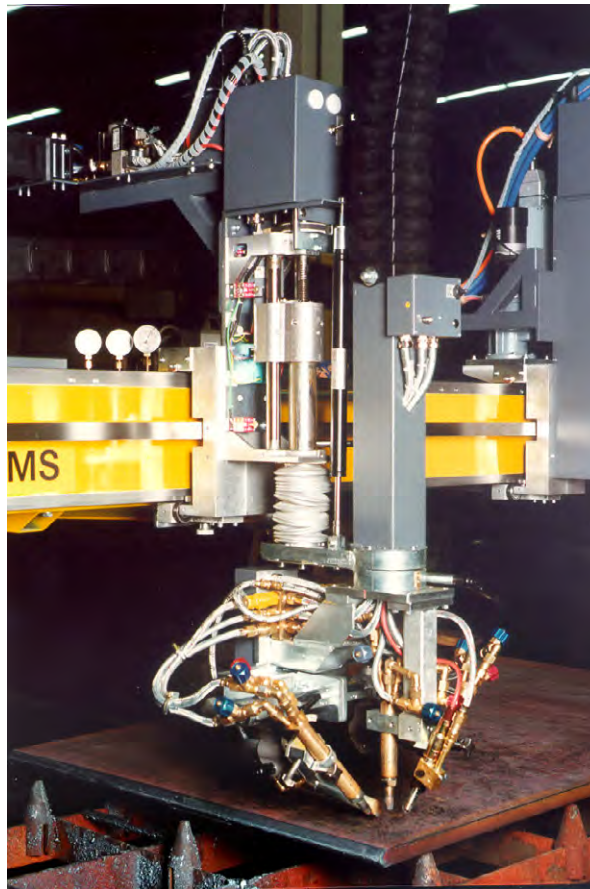
Głowica trójplanikowa, ukosująca MR ± 90° (obrót centralny, nastawy ręczne)
